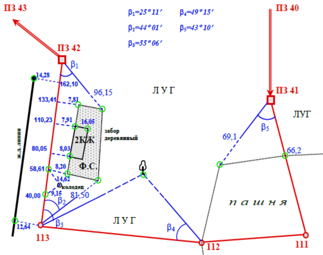
Абрис теодолитной съемки
