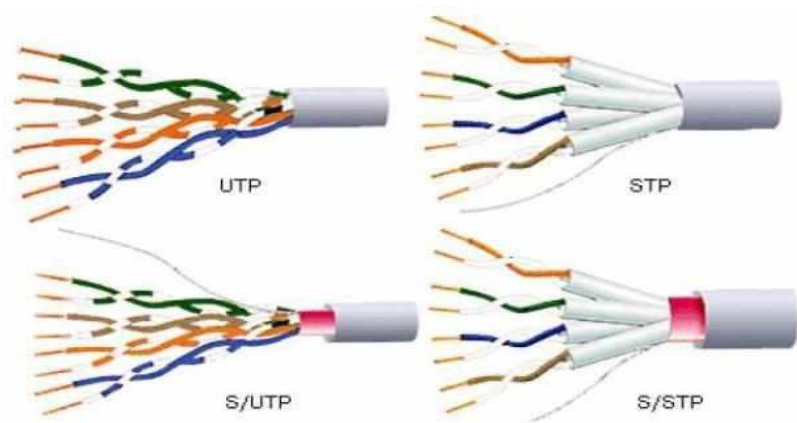
Рисунок 1 – Витая пара
