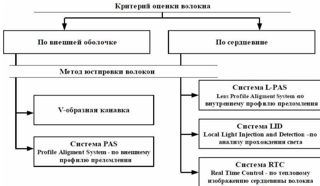
Рисунок 1 – Классификация методов юстировки ОВ
