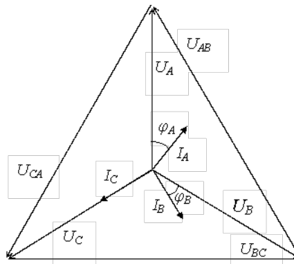
Рис. 1. Векторная диаграмма для трехфазной четырехпроводной схемы при соединении нагрузки «звездой»
